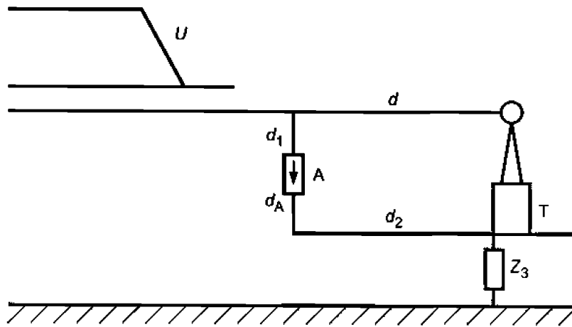
Рисунок 2а — Установки без контура заземления (распределительные сети)
