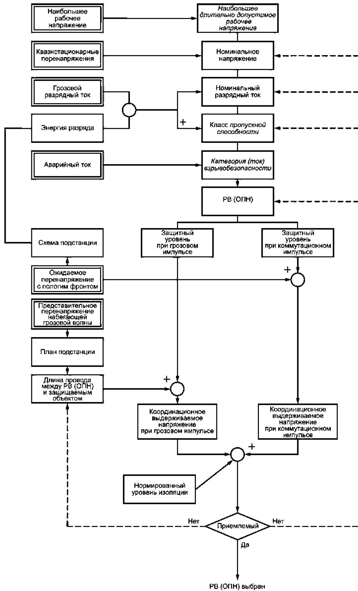
Рисунок 1 — Структурная схема выбора РВ (ОПН)
