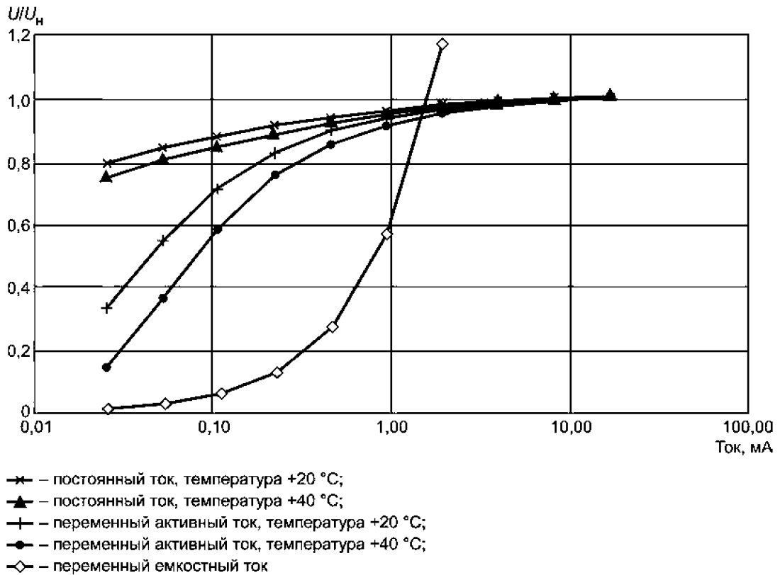
Рисунок 5 — Типичные вольтамперные характеристики нелинейных металлооксидных резисторов
