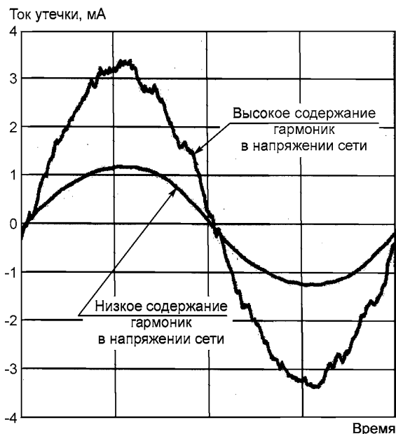
Рисунок 4 — Типичный ток утечки ОПН в условиях эксплуатации
