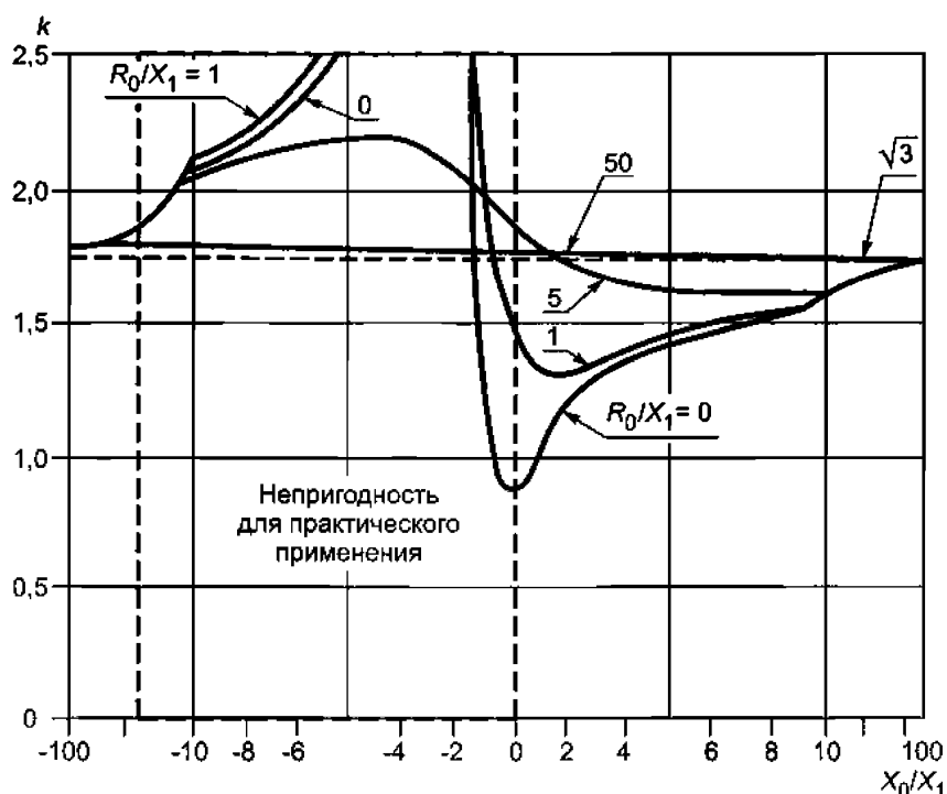
Рисунок А.1 — Коэффициент замыкания на землю k на основе X_0/X_1 , для R_1/X_1 = R = 0
