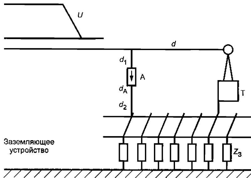
Рисунок 2б — Установки с контуром заземления (подстанции)
