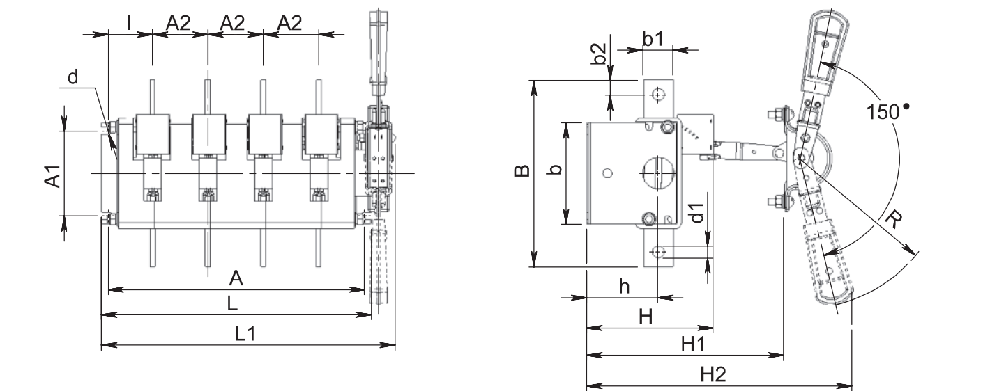
Рис. 21. Выключатель-разъединитель на одно направление 4-полюсный с передней смещенной рукояткой
