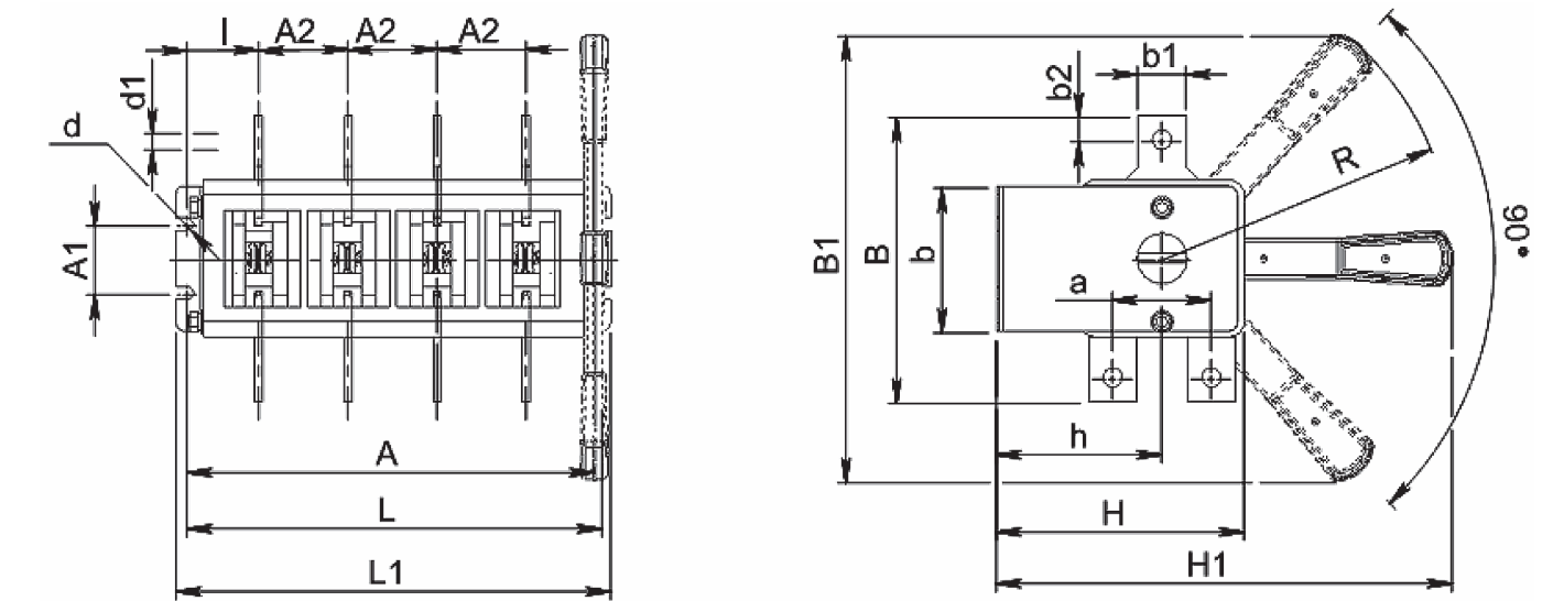
Рис. 22. Выключатель-разъединитель на два направления 4-полюсный с боковой рукояткой
