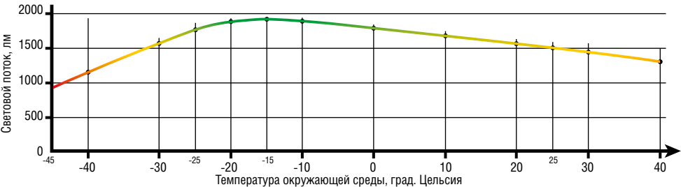
График зависимости светового потока от температуры окружающей среды для лампы Navigator NCL-SH10-28-E27/Outdoor
